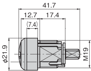
C-466-CG-RK オペレーションキー Operation key
