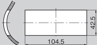
パネル穴明け寸法 Panel drilling dimensions
