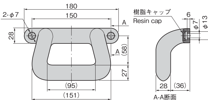
A-A断面 A-Asection
