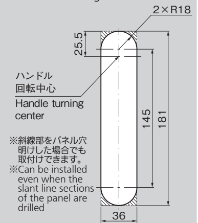
パネル穴明け寸法 Panel drilling dimensions
