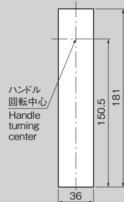
パネル穴明け寸法 Panel drilling dimensions
