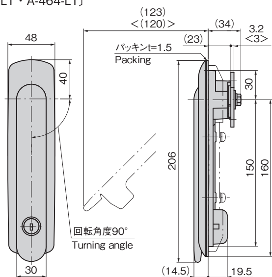
A-464-L1-1
