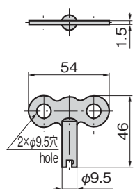
[A-167-H ハンドル] Handle
