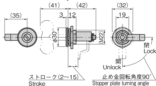
[A-167-2 本体] Main body
