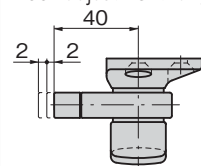
フック調整幅 Hook adjustment range
