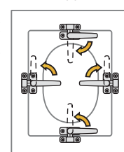
ハンドル固定ねじ Handle fixing screw
