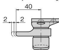
フック調整幅 Hook adjustment range
