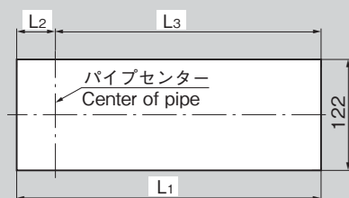
パネル穴明け寸法 Panel drilling dimensions
