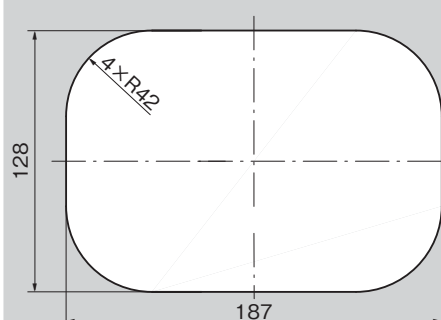
パネル穴明け寸法 Panel drilling dimensions
