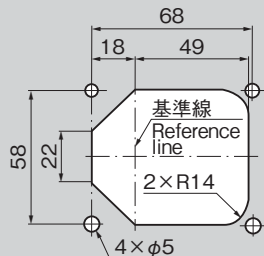
パネル穴明け寸法 Panel drilling dimensions
