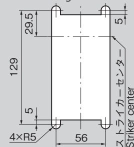
パネル穴明け寸法 Panel drilling dimensions
