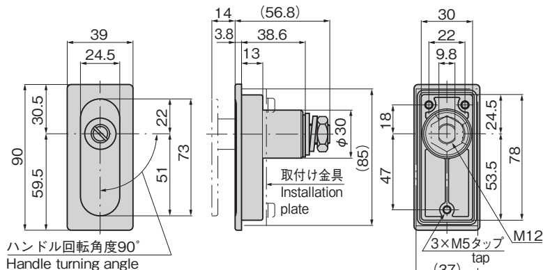
取付け方法 Installation method
