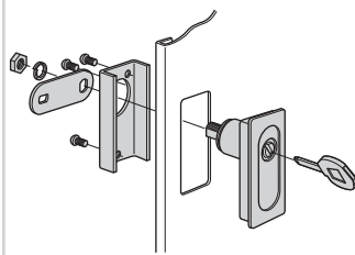
取付け方法 Installation method
