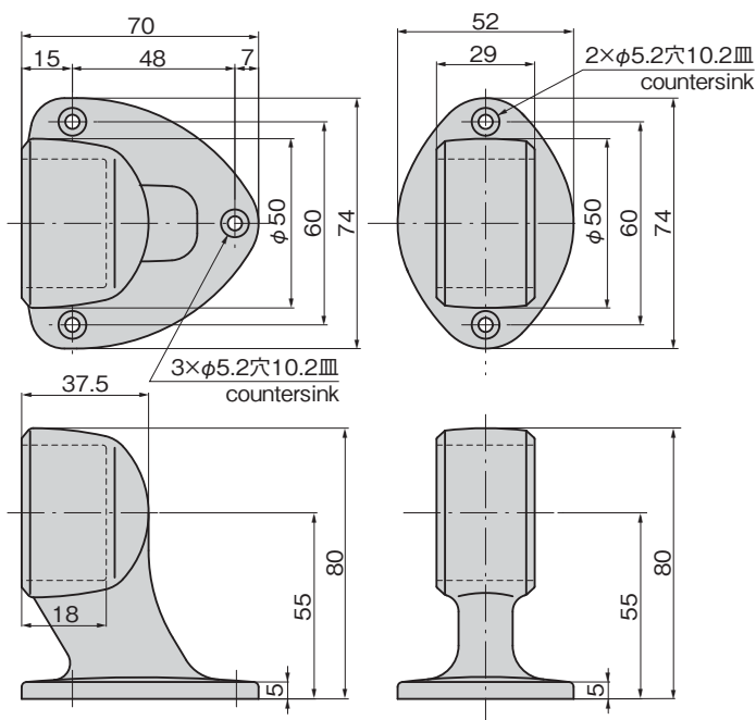
〔A-224-A〕 止め金具 Stopper
