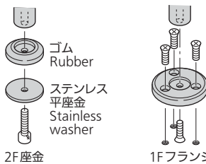
取付け方法 Installation method
