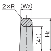
A-A断面図 Cross section A-A
