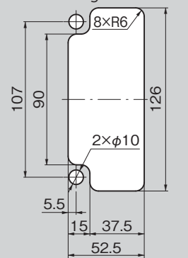
パネル穴明け寸法 Panel drilling dimensions
