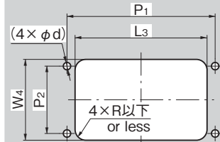
パネル穴明け寸法 Panel drilling dimensions
