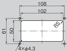
パネル穴明け寸法 Panel drilling dimensions
