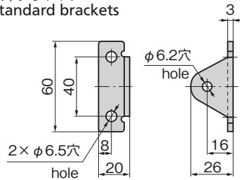
B-461-1用 標準ブラケット Standard brackets
