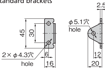
B-461-2~4用 標準ブラケット Standard brackets
