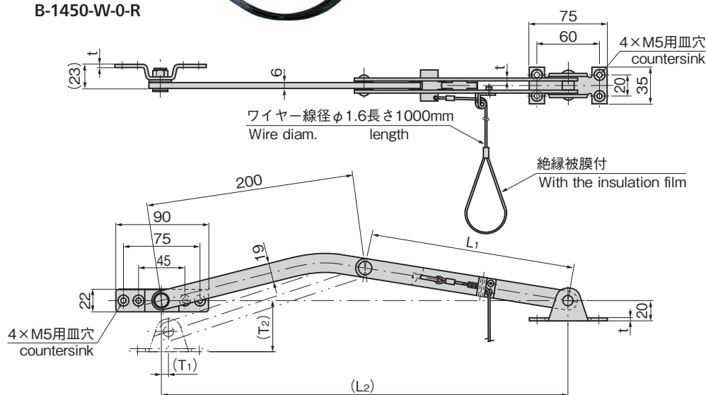
B-1450-W-0-R
