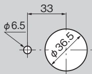
パネル穴明け寸法 Panel drilling dimensions
