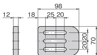
[台座 Spacer]
