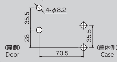
パネル穴明け寸法(C-1567-R) Panel drilling dimensions
