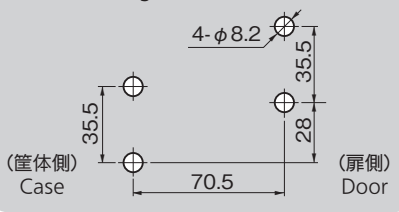
パネル穴明け寸法(C-1567-L) Panel drilling dimensions
