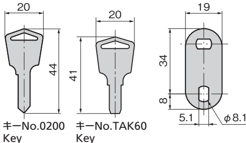
キーNo. 0200 Key
