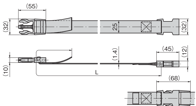
バックル接合図 Buckling diagram
