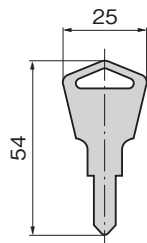
キーNo. T0230 Key
