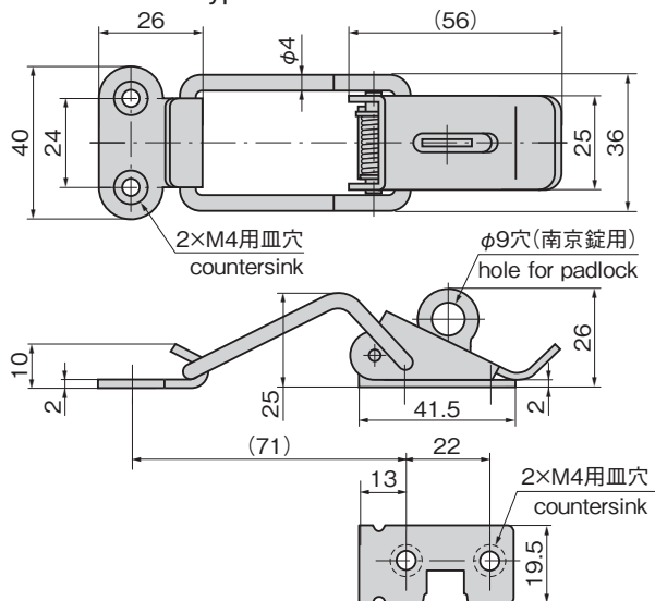
〔C-1142-1〕 (フラットタイプ) Flat type
