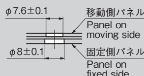
パネル穴明け寸法 Panel drilling dimensions
