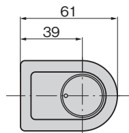
パネル穴明け寸法 Panel drilling dimensions
