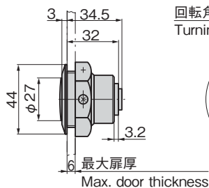
オープン時 When opening
