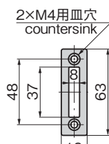
受座 Striker
