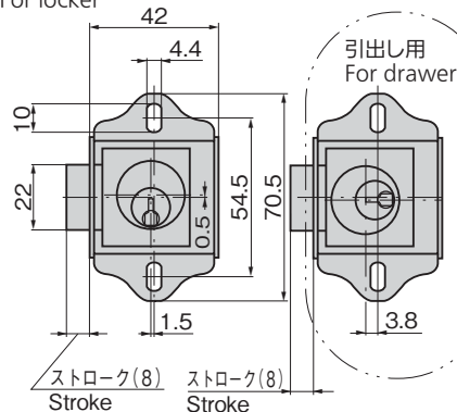
〔C-4-1〕 ロッカー用 For locker
