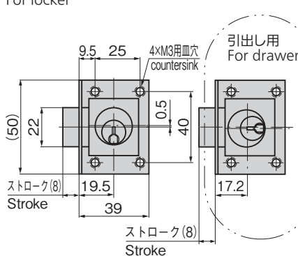
〔C-4-2〕 ロッカー用 For locker
