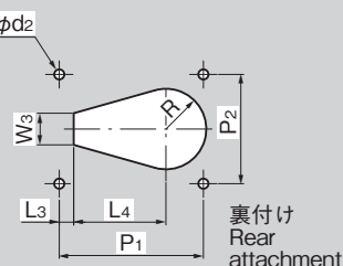
パネル穴明け寸法 Panel drilling dimensions
