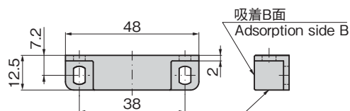
C-185-A [本体 Main body]
