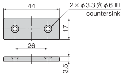
〔受 板 Catch plate〕
