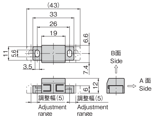
〔本 体 Main body〕
