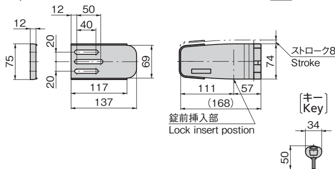
[台座 Spacer]
