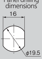
パネル穴明け寸法 Panel drilling dimensions
