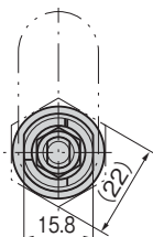
パネル穴明け寸法 Panel drilling dimensions
