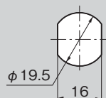
パネル穴明け寸法 Panel drilling dimensions
