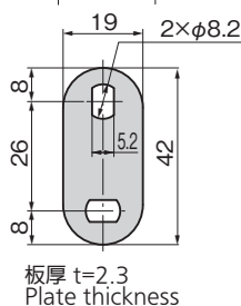
パネル穴明け寸法 Panel drilling dimensions
