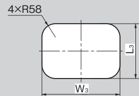
パネル穴明け寸法 Panel drilling dimensions
