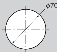
パネル穴明け寸法 Panel drilling dimensions
