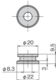
M8用ワッシャー washer
