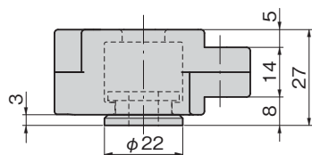
M8用ワッシャー washer
