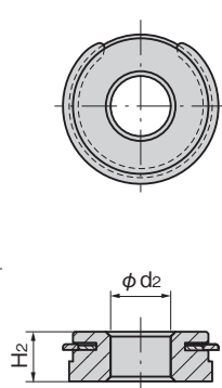
〔座金側〕 Washer
