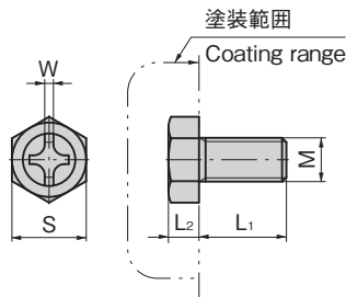
C-209CS-M6×15 〔プラスマイナスタイプ〕 Phillips-standard-head screw
