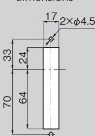
パネル穴明け寸法 Panel drilling dimensions
