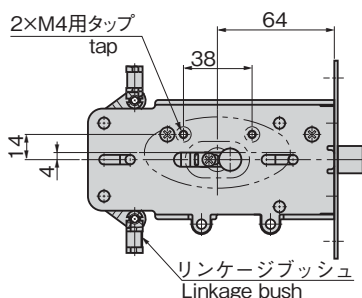
(室外側) (outdoor side) 詳細は1306ページを参照。 See page 1306.
