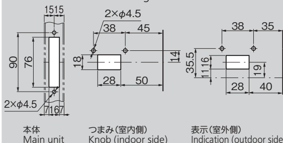
パネル穴明け寸法 Panel drilling dimensions
