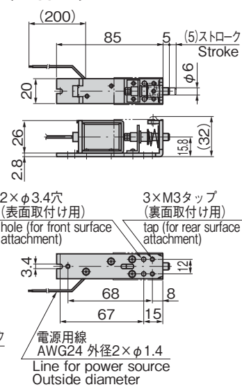
[LE-33-12]
