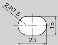
パネル穴明け寸法 Panel drilling dimension
