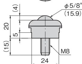
水抜き穴 Drainage hole
