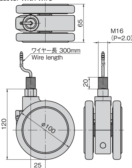
〔ワイヤー付キャスター〕 Caster with wire
