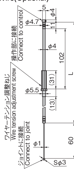
〔ワイヤー(別売)〕 Wire (Optional)
