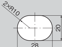
パネル穴明け寸法 Panel drilling dimension
