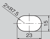
パネル穴明け寸法 Panel drilling dimension
