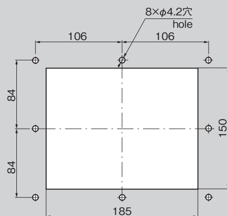
パネル穴明け寸法 Panel drilling dimensions
